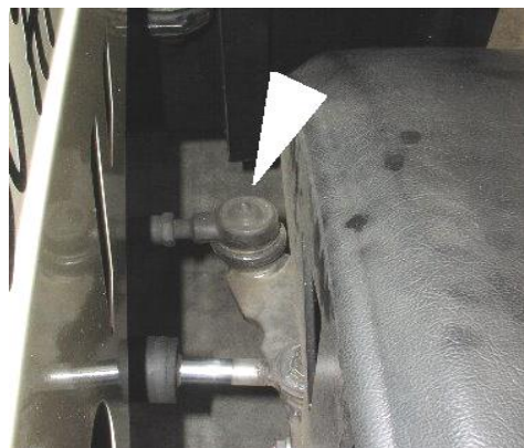
maznice kloubu spojovací tyče (2x)
