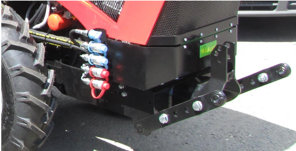
Vývody rychlospojek u předního TBZ
