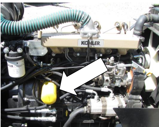
Filtr motorového oleje – mění se celý filtr motor Kohler
