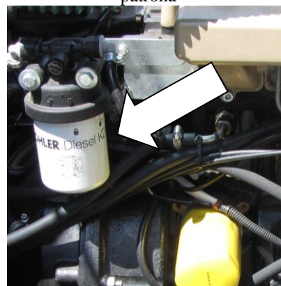
palivový filtr – mění se celá patrona motor Kohler
