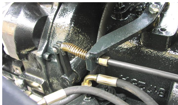
stavěcí šroub s matkou za páčkou spojkového ložiska
