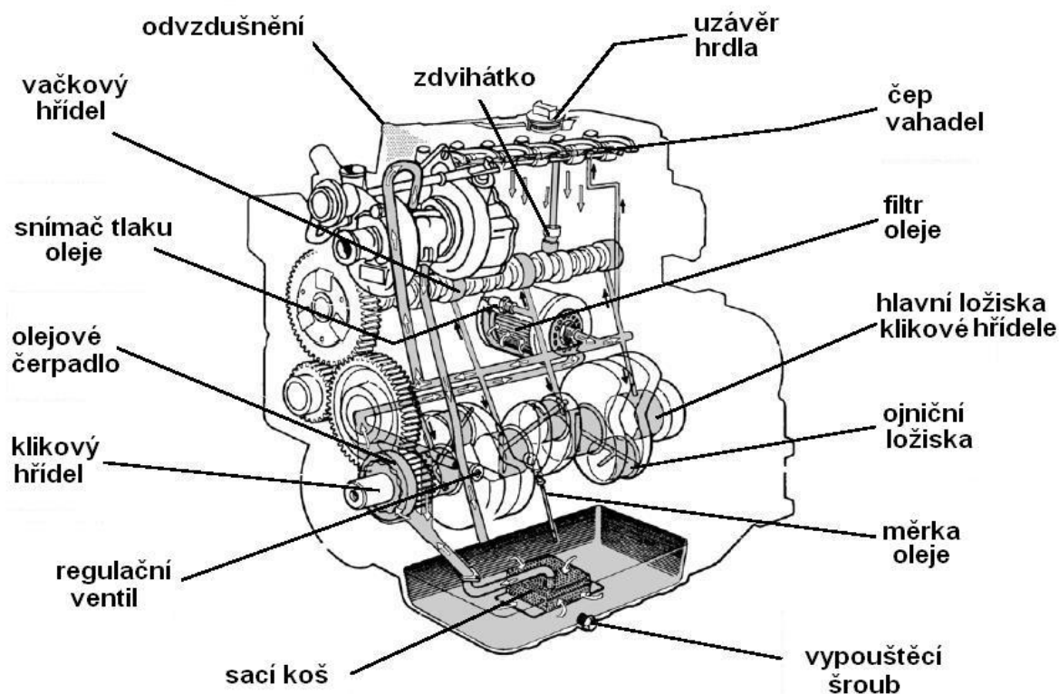
Schéma mazání
