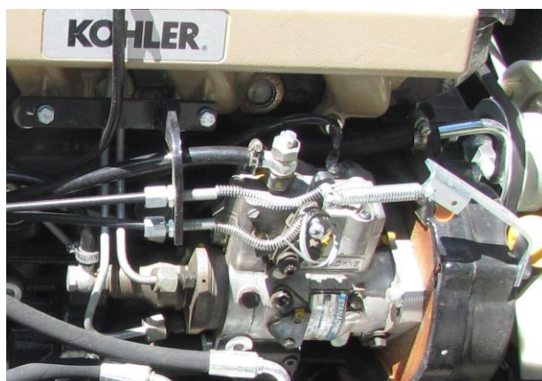
Horní lanko řídí otáčky, dolní startovací dávku , motor Kohler
