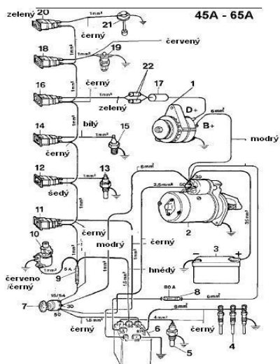
schéma napájecího obvodu elektriky u motorů
