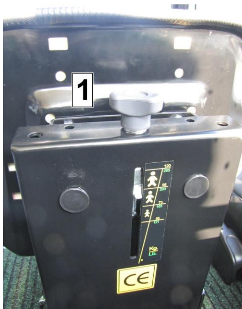
svislé nastavení sedačky
